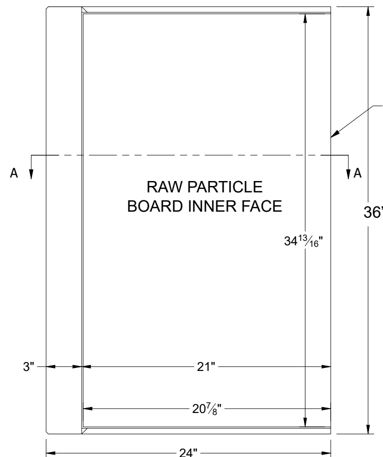
4 31 ELEVATION
